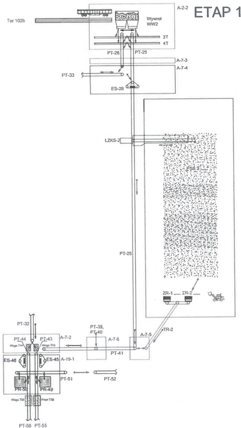
Rys. 4.3 - Schemat poglądowy ciągu transportowego od wywrotnicy WW2, budynek A-2-2, poprzez taśmociągi 3T1, 3T2, 4T1, 4T2, PT-25, PT-26, budynek A-7-3, A-7-4 z urządzeniami, ładowarko - zwałowarkę ŁZKS-2, budynek A-7-5, nowoprojektowanym taśmociągłem TR-2 (500m 3 /h) A-7-6, PT-41, PT-43, PT-44, PT-51, PT-55, PT-56,
